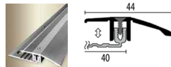
486 2-teiliges Anpassungsprofil
