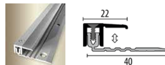
487 2-teiliges Abschlussprofil
