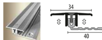
488 2-teiliges Übergangprofil
