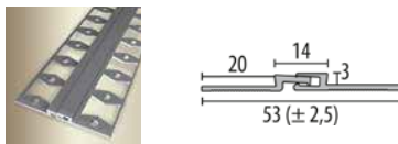
317 Bewegungsfugenprofil
