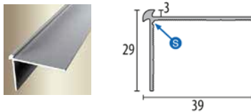
871 Treppenkantenprofil
