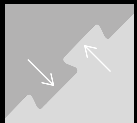
Schwalbenschwanzverbindung
