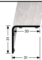
AUSSENWINKEL EXTERIOR ANGLE
