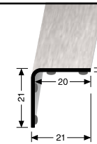
AUSSENWINKEL EXTERIOR ANGLE
