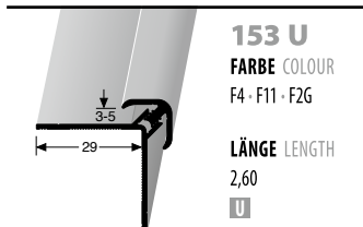
2-TEILIGE CLIP-AUSSENECKE 2-PART CLIP EXTERIOR CORNER
